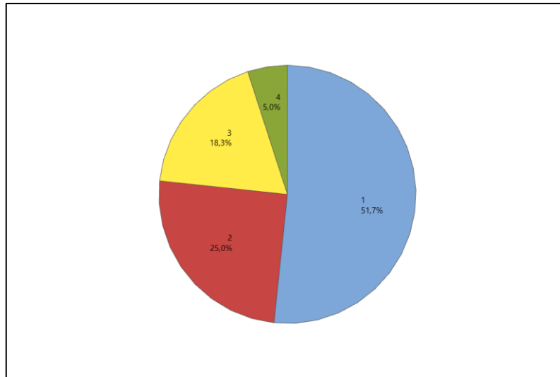
Gambar 4. Pie Chart Tipe Mobil
