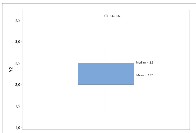
Gambar 3. Boxplot Kapasitas Mesin Mobil
